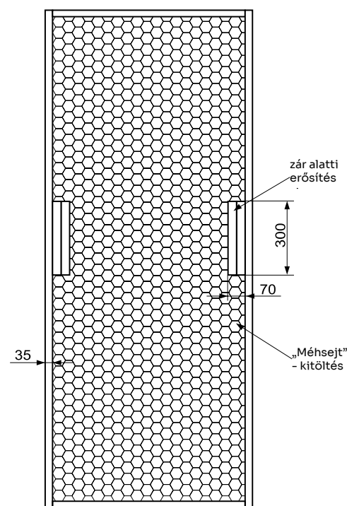
Lemezelt ajtószárny felépítése
