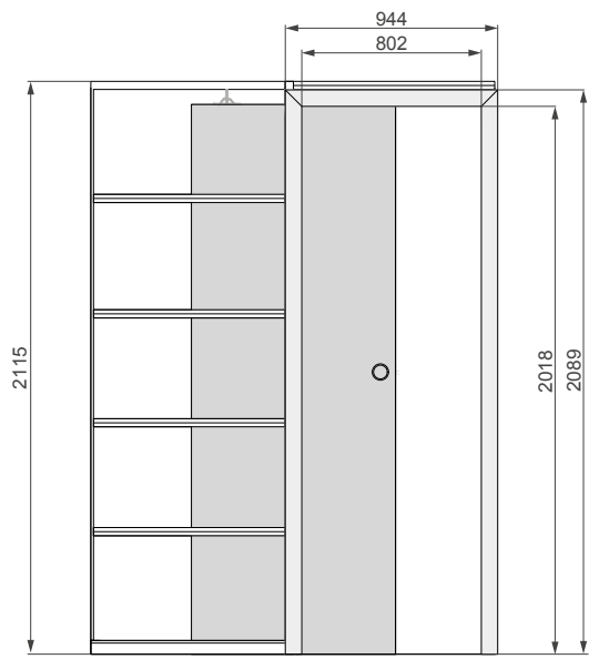
Beépítés G/K rendszerbe: 60 mm-es takaróléc
