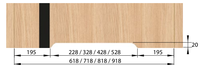
Szellőző-kivágás a MODERNO, LAMELO, MAGNETIC L, INTARSJA 40 ajtószárnyakban
