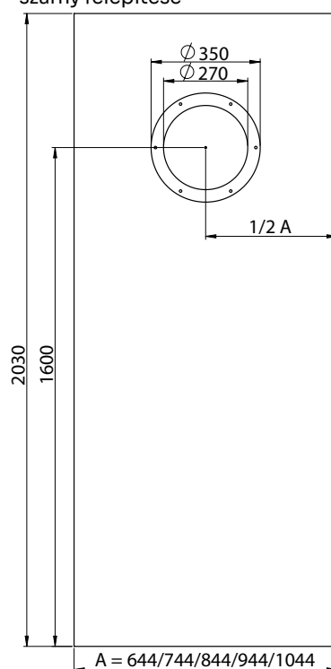
BULAJ falcos szárny felépítése
