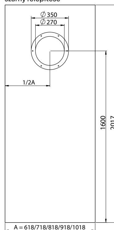
BULAJ falc nélküli szárny felépítése
