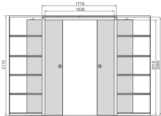
KETTŐS G/K KAZETTA ajtószárnyak
